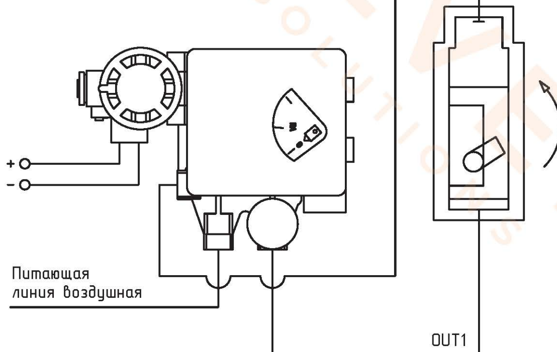
Рисунок 8 – Схема подключения пневматических сигналов для привода обратного действия.
