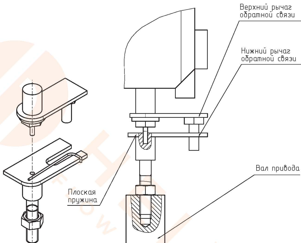
Рисунок 3 – Схема соединения позиционера с пневмоприводом.
