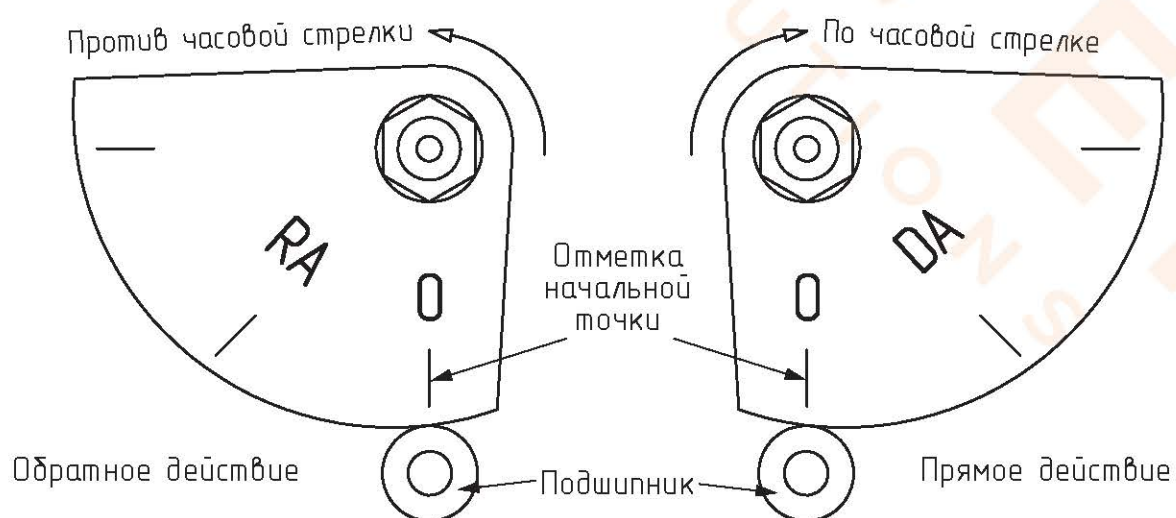
Рисунок 4 – Установка шкалы положения.
