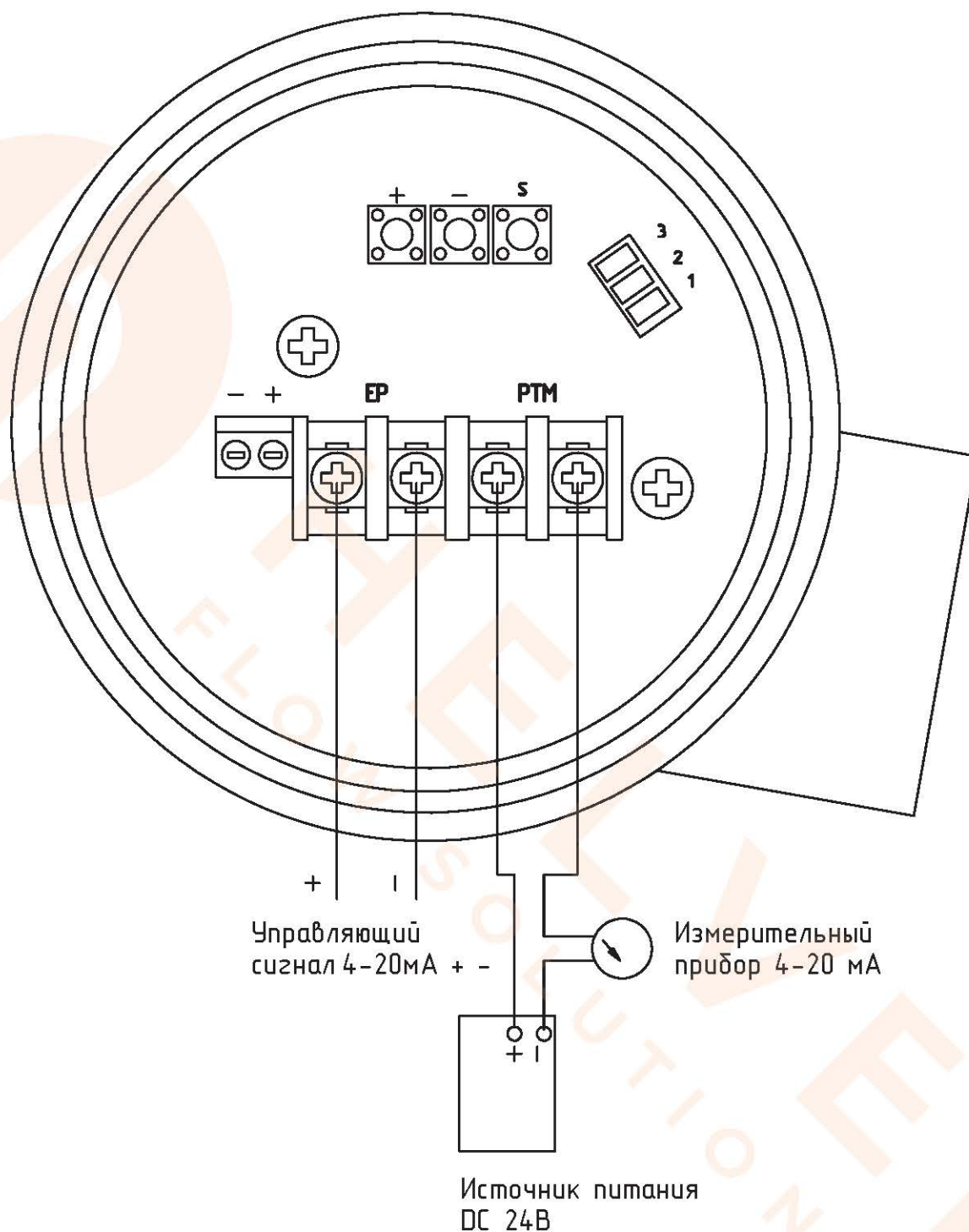
Рисунок 6 – Схема подключения электрических сигналов EPP-R-2.
