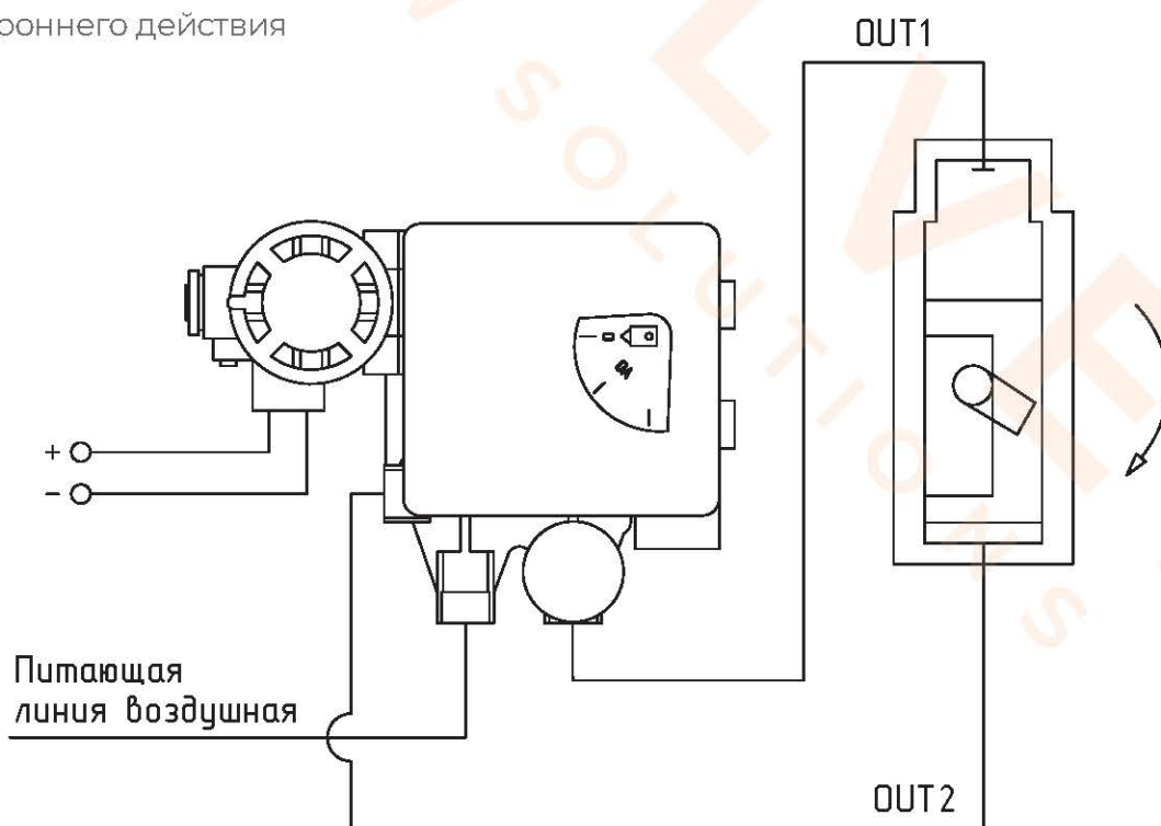
Рисунок 7 – Схема подключения пневматических сигналов для привода прямого действия.
